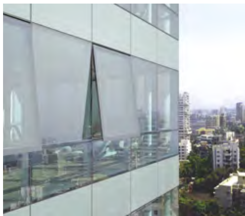
Schüco TropTec UC 65 SG.NI with Schüco TropTec AW 58.NI insert unit Schüco TropTec UC 65 SG.NI mit Schüco TropTec AW 58.NI Einseitzelement
