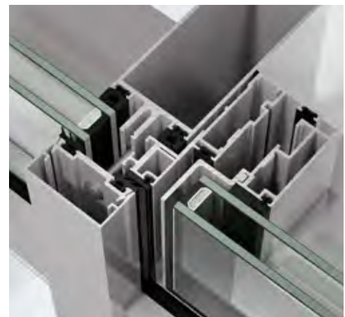
Schüco TropTec AW 58.NI in Schüco TropTec SC 50.NI with double glazing Schüco TropTec AW 58.NI in Schüco TropTec SC 50.NI mit Isolierverglasung
